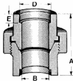
VR1526 Assento Integral
